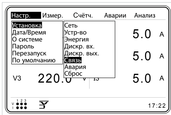
Рис. 3-44 Меню Связь
