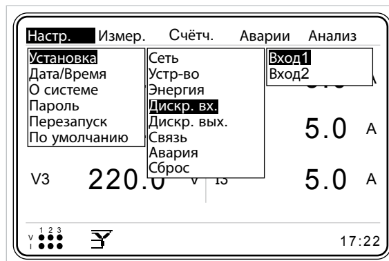
Рис. 3-28 Меню Дискр. вх.
