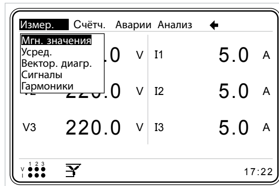
Рис. 3-67 Меню Измерения
