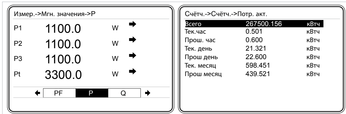
Рис. 3-69 Вид экрана при правильном подключении проводников K-L трансформатора тока
