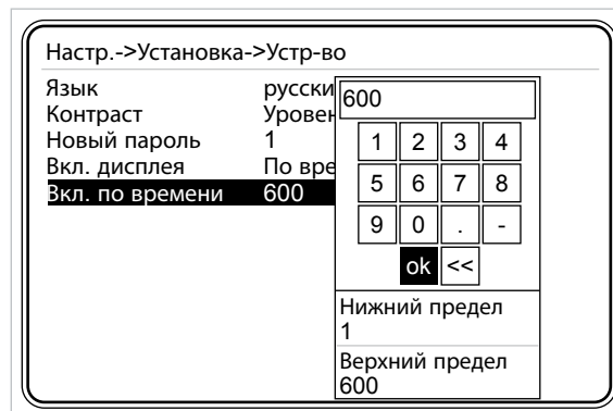
Рис. 3-23 Выбор времени подсветки дисплея
