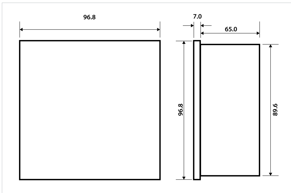
Рис. 2-9 Размеры
