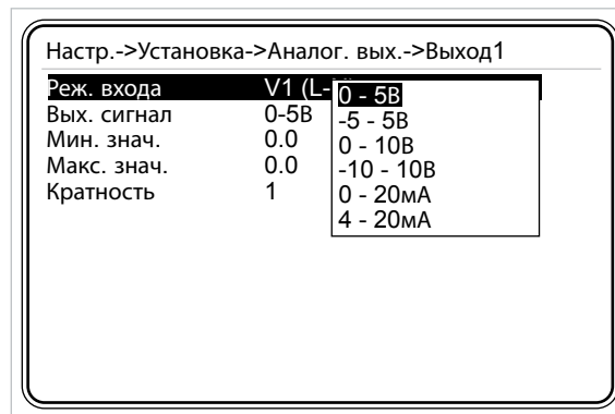
Рис. 3-40 Подменю Вых. сигнал
