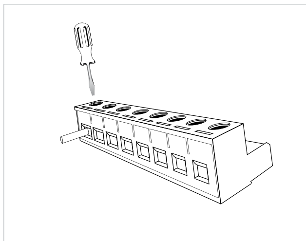
Рис. 2-5 Фиксация кабеля винтовым зажимом клеммного блока
