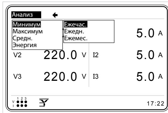
Рис. 3-94 Меню Минимум
