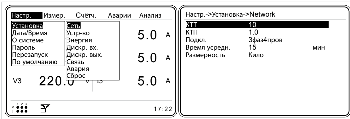
Рис. 3-13 Меню Сеть
