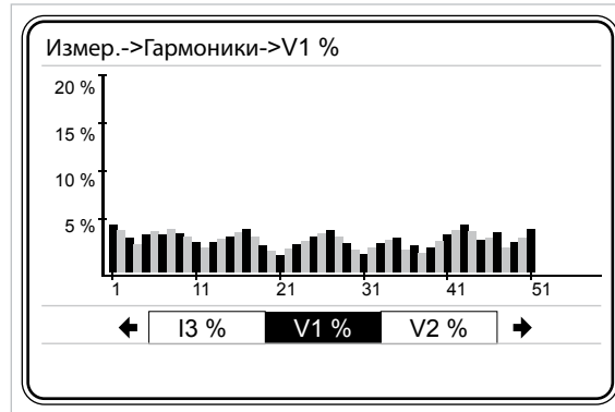
Рис. 3-79 Отображение гармоник в виде графика
