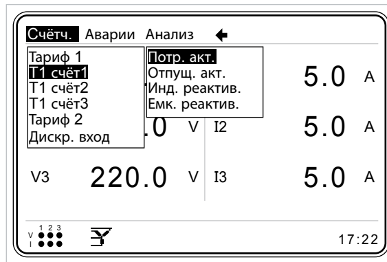
Рис. 3-85 Меню T1 счёт1
