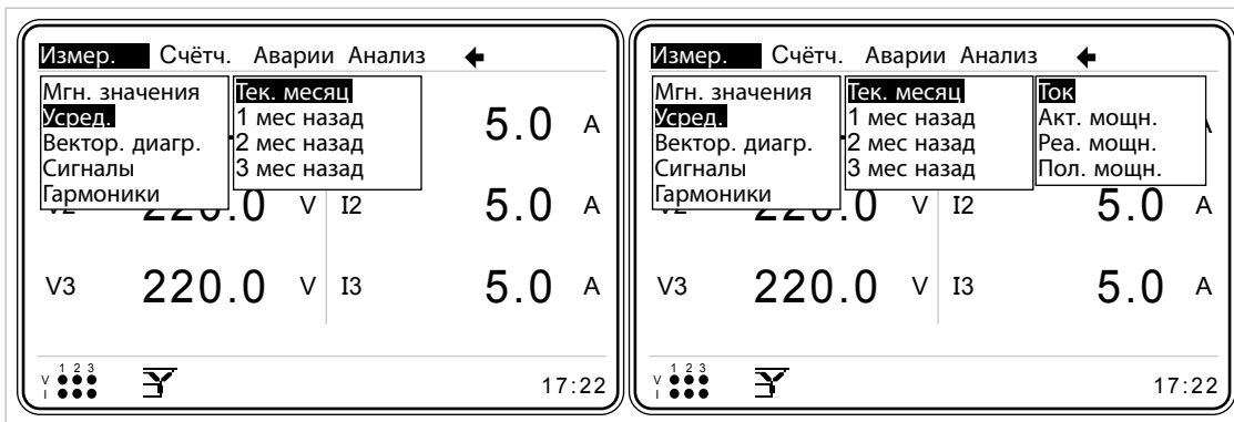
Рис. 3-72 Меню Тек. месяц
