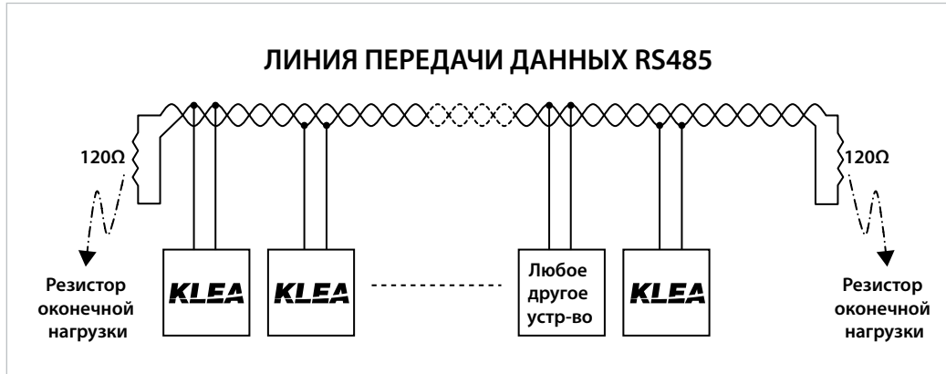
Рис. 4-1 Схема подключения к линии RS485
