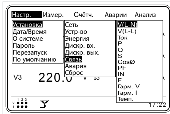
Рис. 3-47 Подменю Авария
