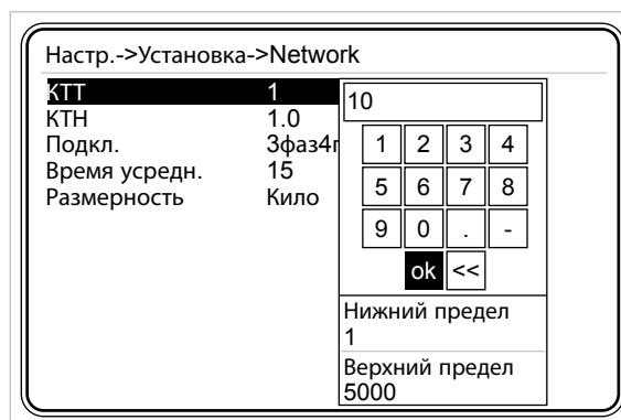
Рис. 3-14 Настройка коэффициента трансформации ТТ
