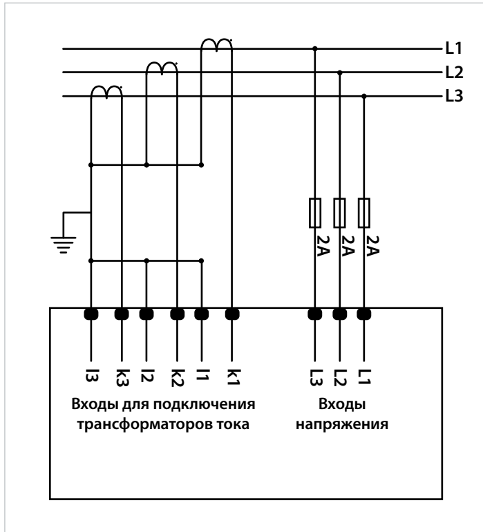
Рис. 2-7 Трёхфазное подключение анализатора KLEA по схеме "треугольник"
