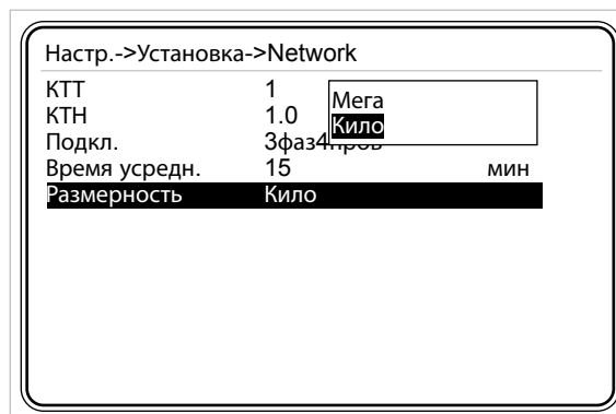
Рис. 3-18 Выбор размерности показаний
