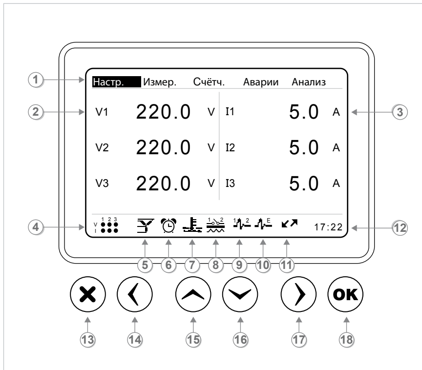
Рис. 1-1 Дисплей KLEA
