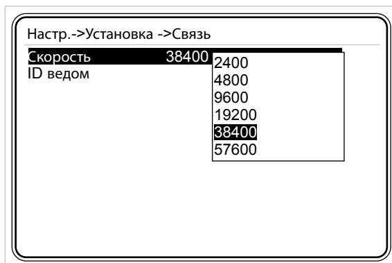
Рис. 3-45 Настройка скорости передачи данных
