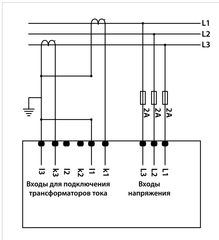
Рис. 2-8 Подключение анализатора KLEA по схеме Арона
