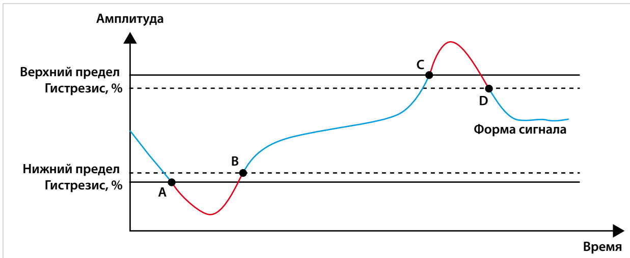
Рис. 3-52 Пример срабатывания аварийной сигнализации
