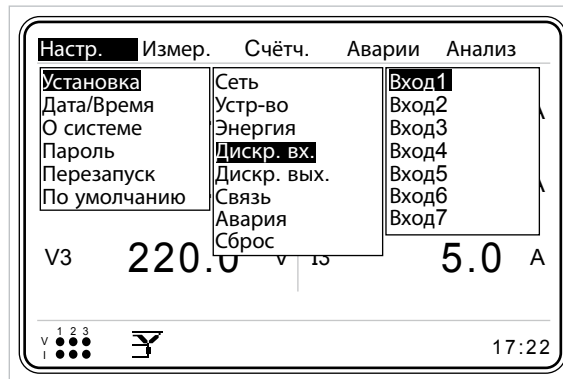
Рис. 3-29 Меню анализатор с дополнительными входами и выходами
