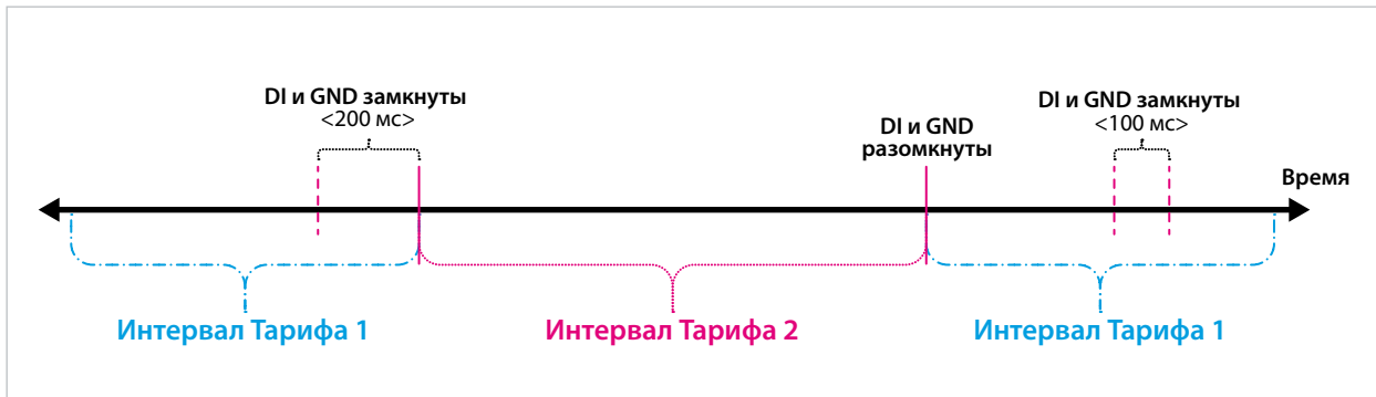
Рис. 3-33 Активация подсчёта по Тарифу 1 и Тарифу 2
