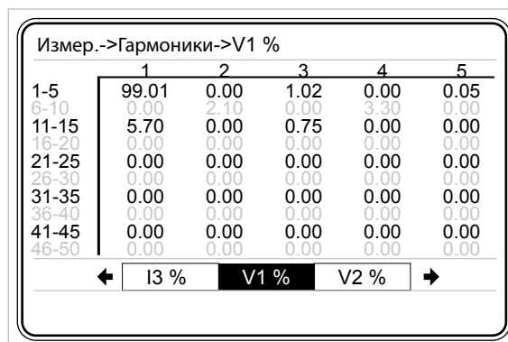
Рис. 3-78 Отображение гармоник в виде таблицы
