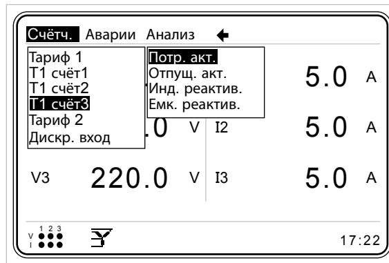
Рис. 3-87 Меню T1 счёт3
