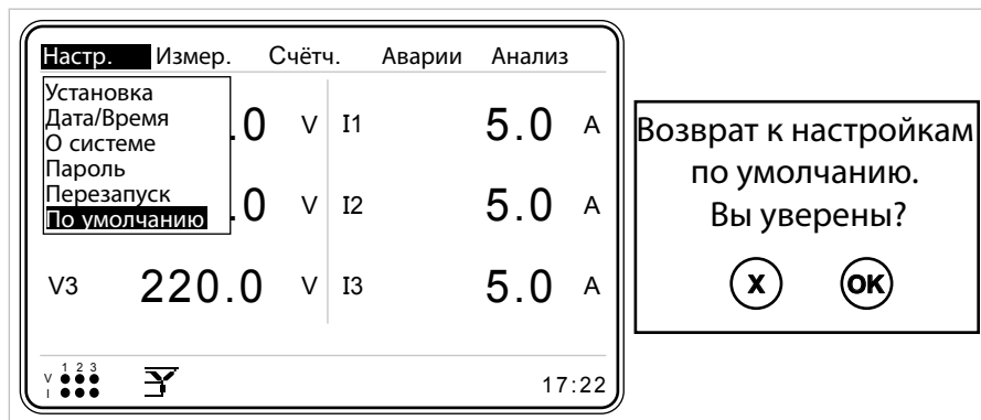
Рис. 3-66 Команда "По умолчанию"
