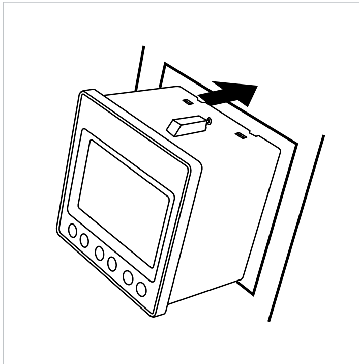
Рис. 2-1 Монтаж KLEA в вырезе панели
