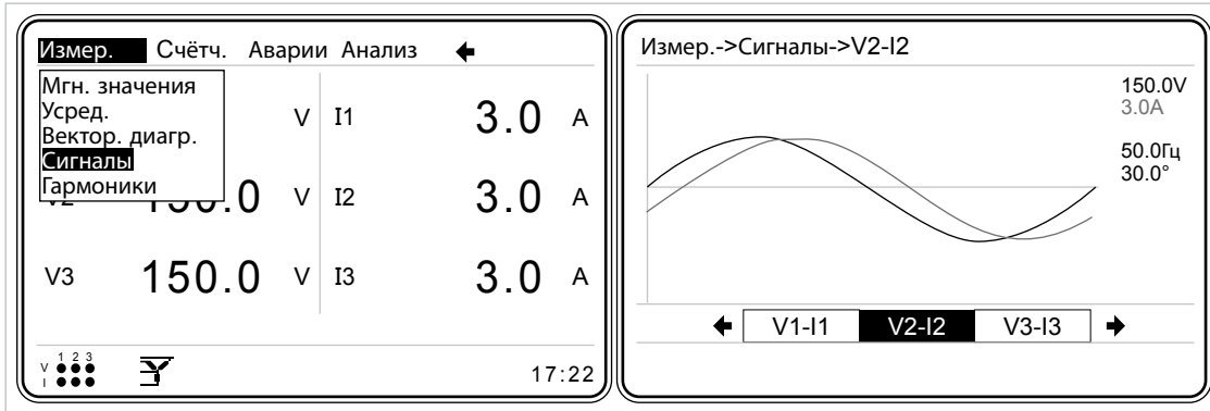
Рис. 3-76 Меню Сигналы
