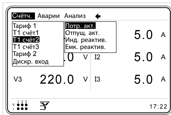
Рис. 3-86 Меню T2 счёт2
