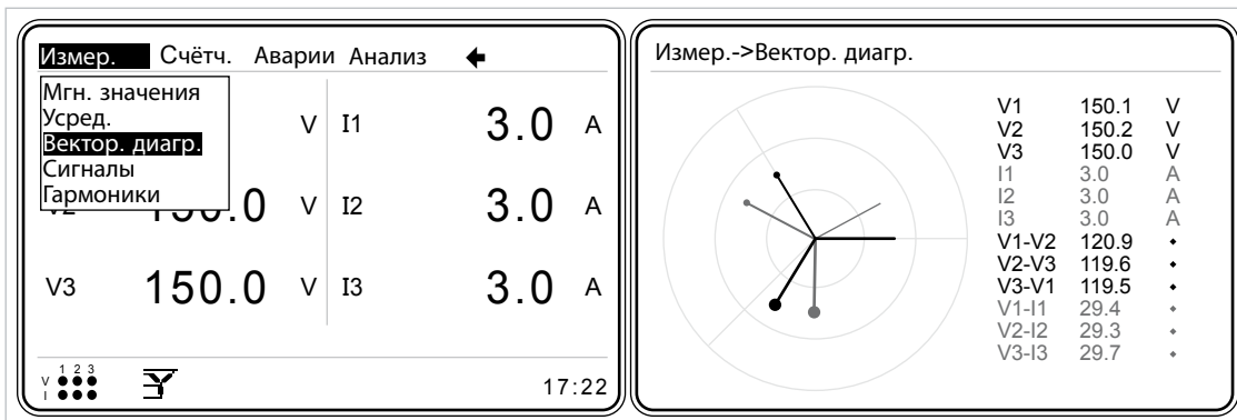
Рис. 3-75 Меню Вектор. диагр.
