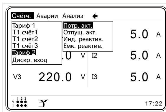
Рис. 3-88 Меню Тариф 2
