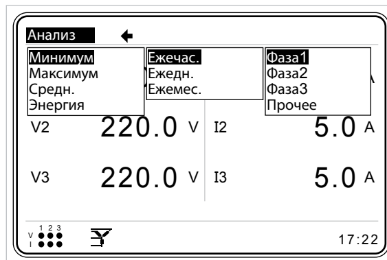
Рис. 3-95 Меню Ежечас.
