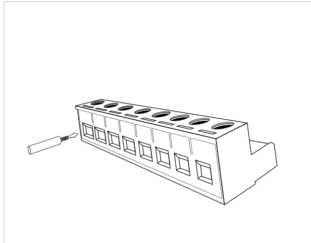
Рис. 2-4 Подключение кабеля к клеммному блоку
