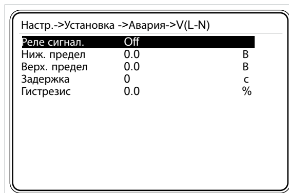
Рис. 3-48 Подменю V(L-N) – фазное напряжение
